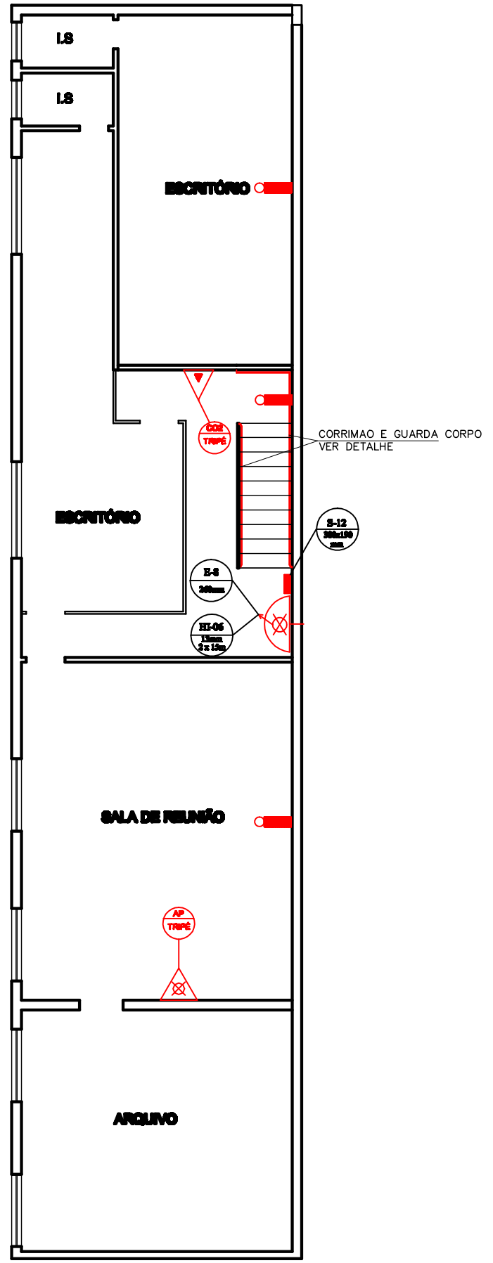
PLANTA 2º PAVTO GALPÃO 2 ESC. 1/50 ÁREA: 157,20 m²
