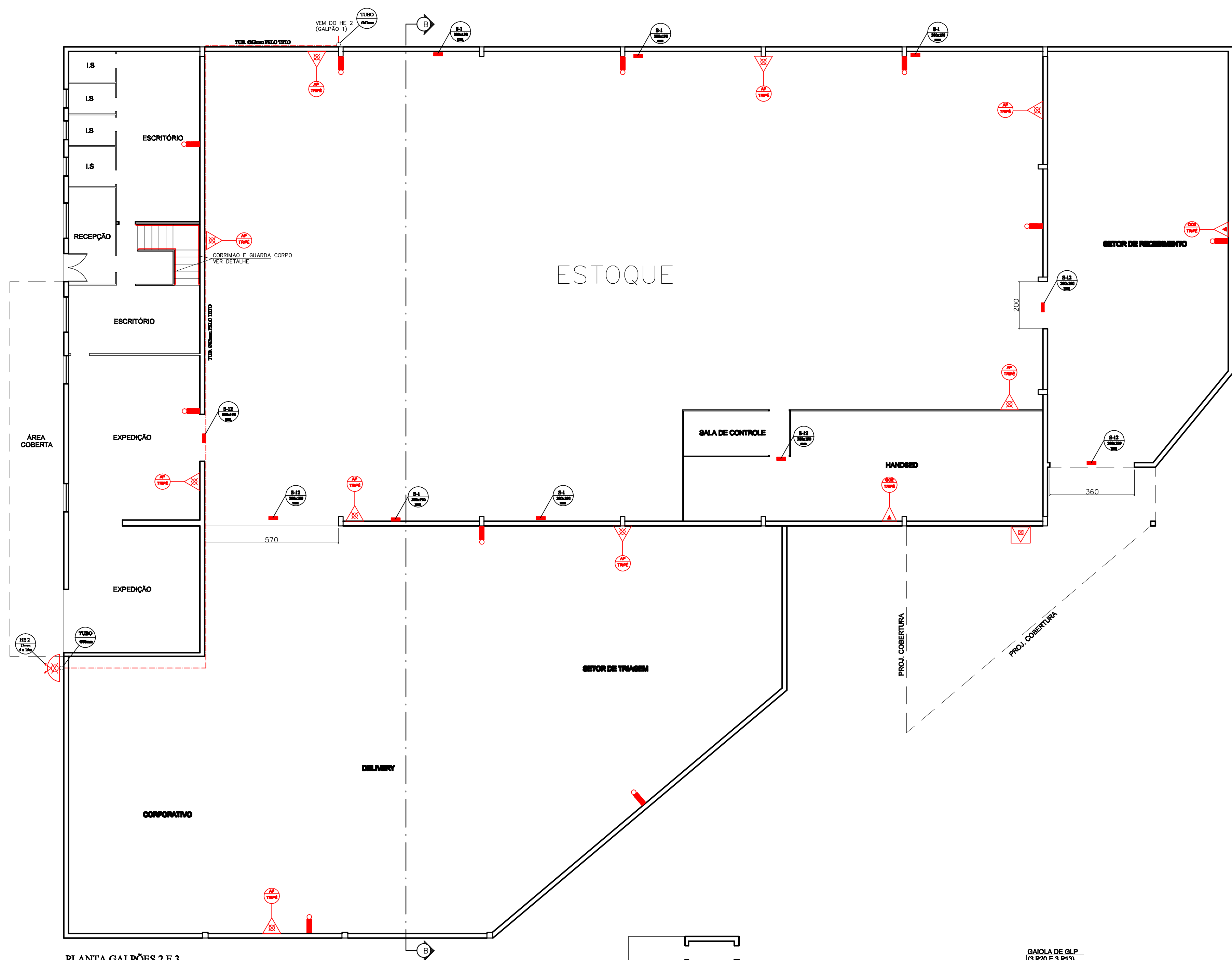
PLANTA GALPÕES 2 E 3 ESC. 1/50 ÁREA: 1.569,54 m²
