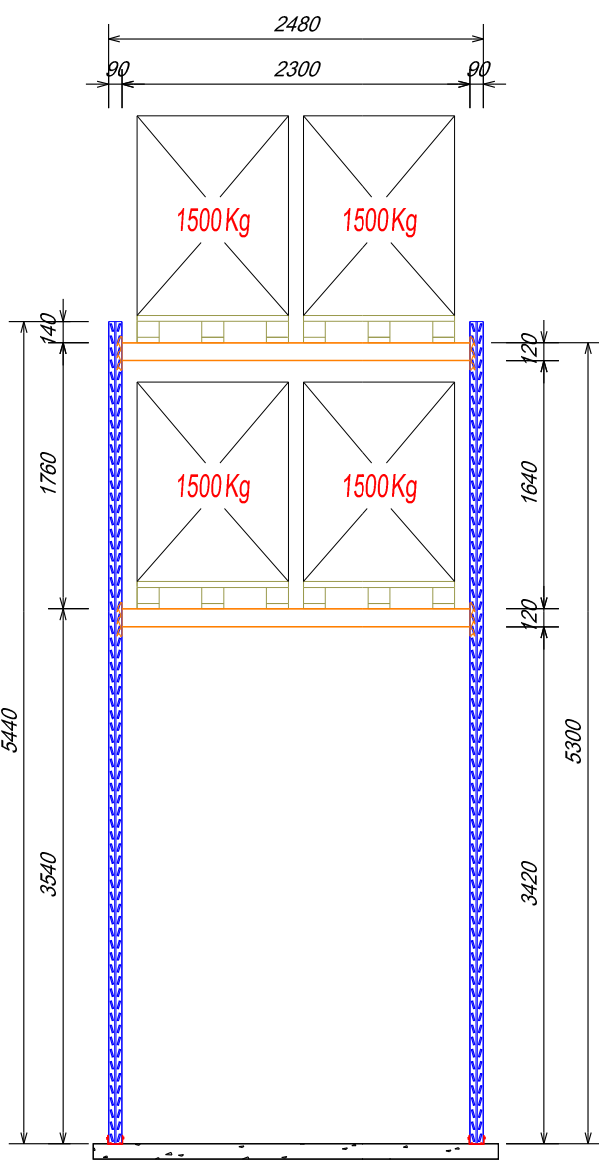
VISTA FRONTAL "TÚNEL" ESCALA 1/50
