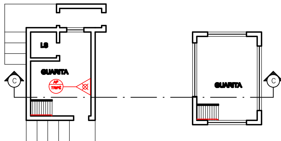
GUARITA 1º PAVTO ESC. 1/50 ÁREA: 13,11 m²
