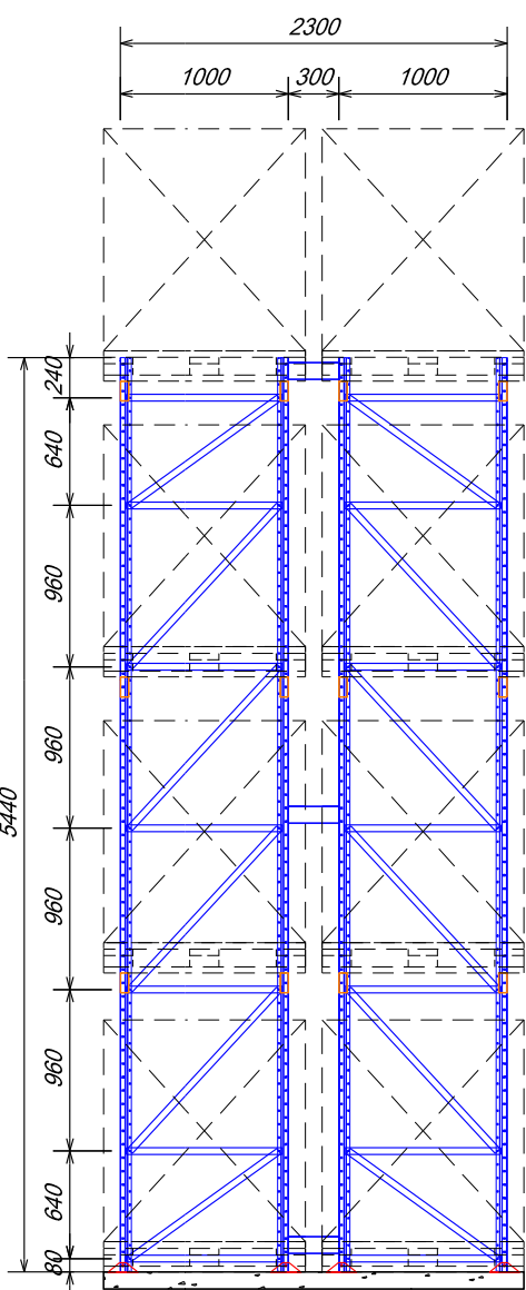
VISTA LATERAL "A" ESCALA 1/50
