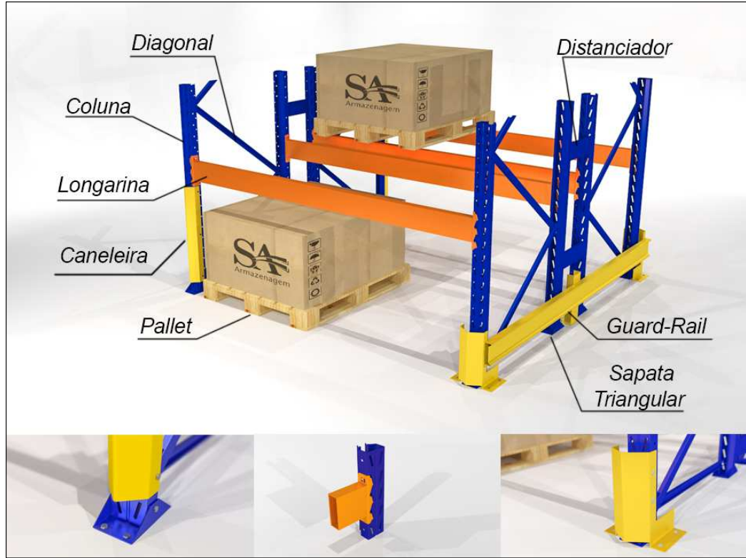
DETALHE PORTA PALLETS (ILUSTRATIVO)
