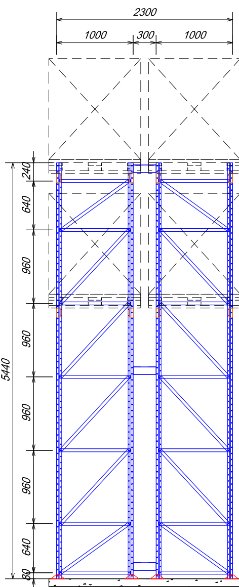
VISTA LATERAL "TÚNEL" ESCALA 1/50
