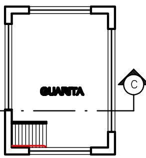
GUARITA 2º PAVTO ESC. 1/50 ÁREA: 10,92 m²
